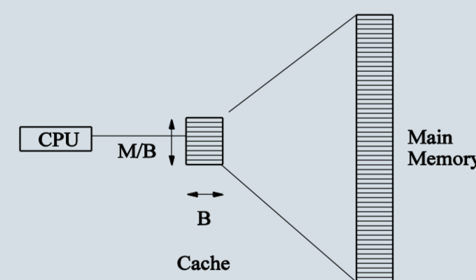
EM model
